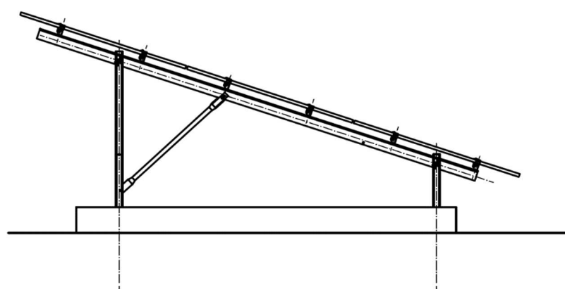
Figure 12 : Schéma de principe des fixations avec plots bétons (Source : Axial)
