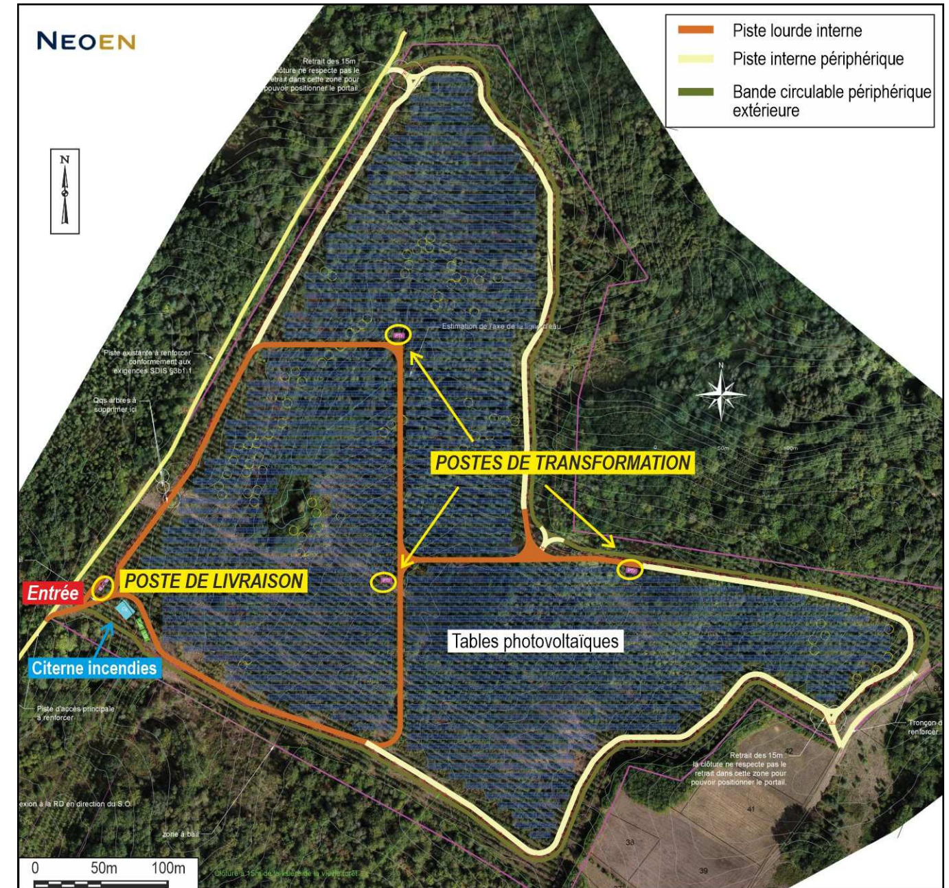
Figure 76 : Localisation des pistes et aménagements
