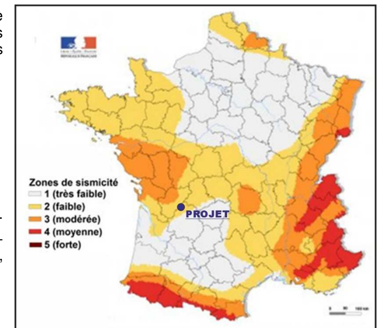
Illustration 19 : Zonage sismique
