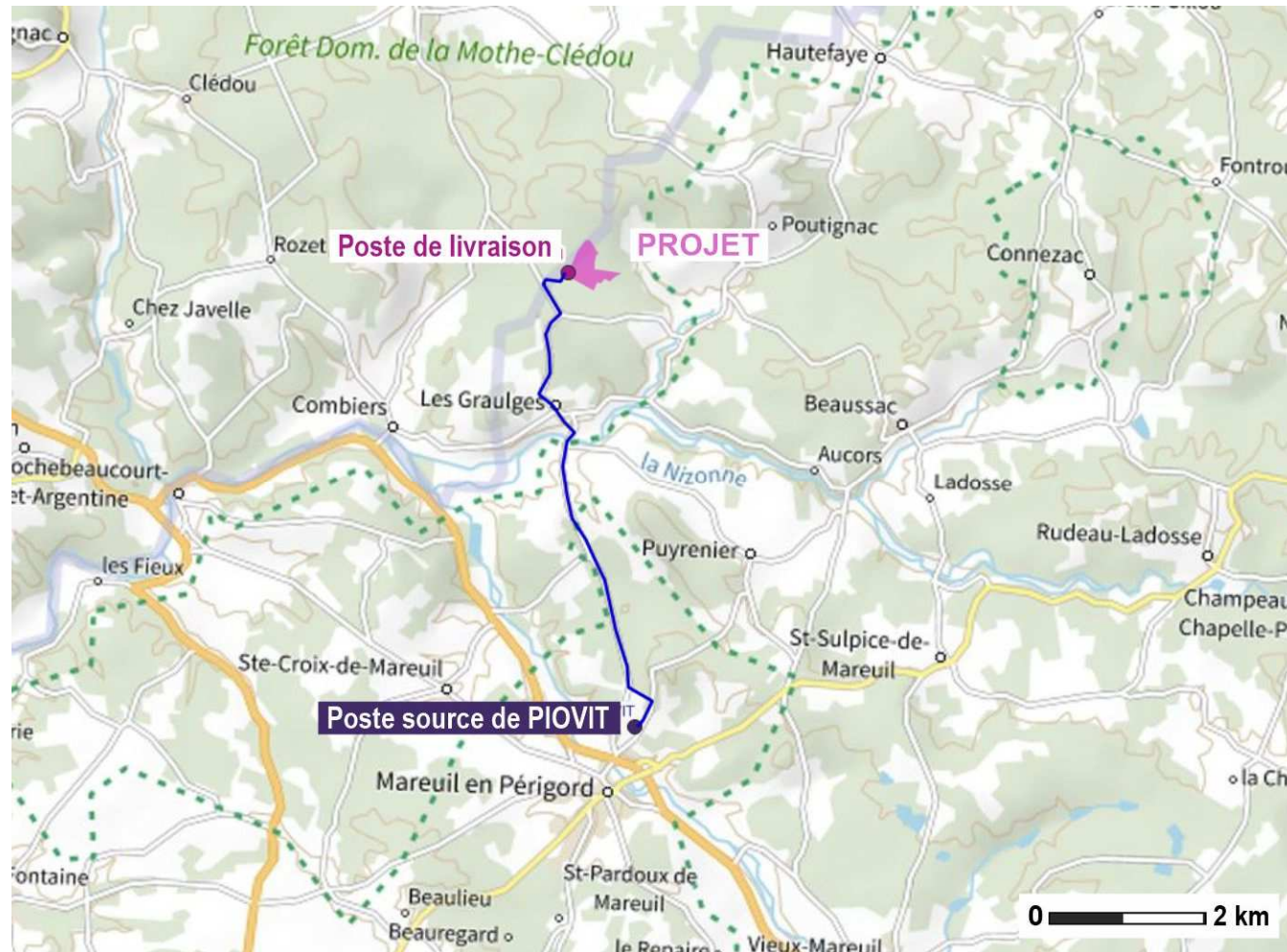
Figure 13 : Emplacement du poste-source envisagé pour le raccordement électrique du projet
