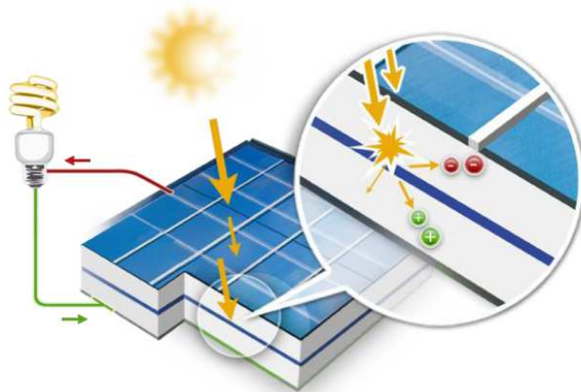
Figure 9 : Schéma de principe de l'effet photovoltaïque utilisé sur un module photovoltaïque. Source : www.photovoltaique.info
