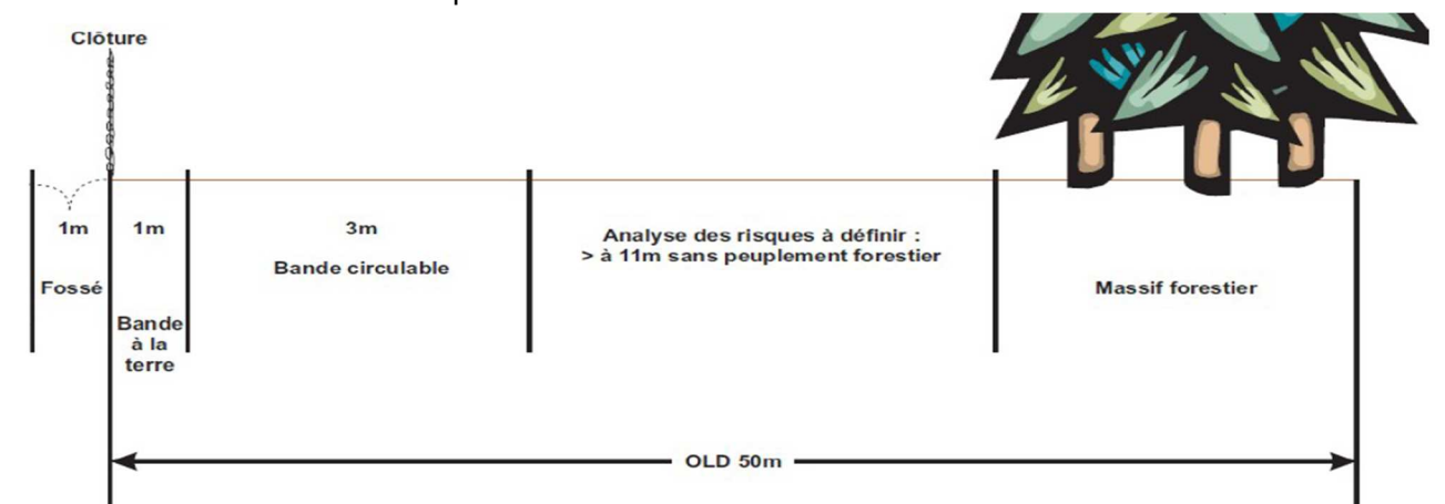
Figure 14 : Principe d'aménagement périphérique du site – Source : « Préconisations pour les parcs photovoltaïques au sol – SDIS 24 - 2022 »
