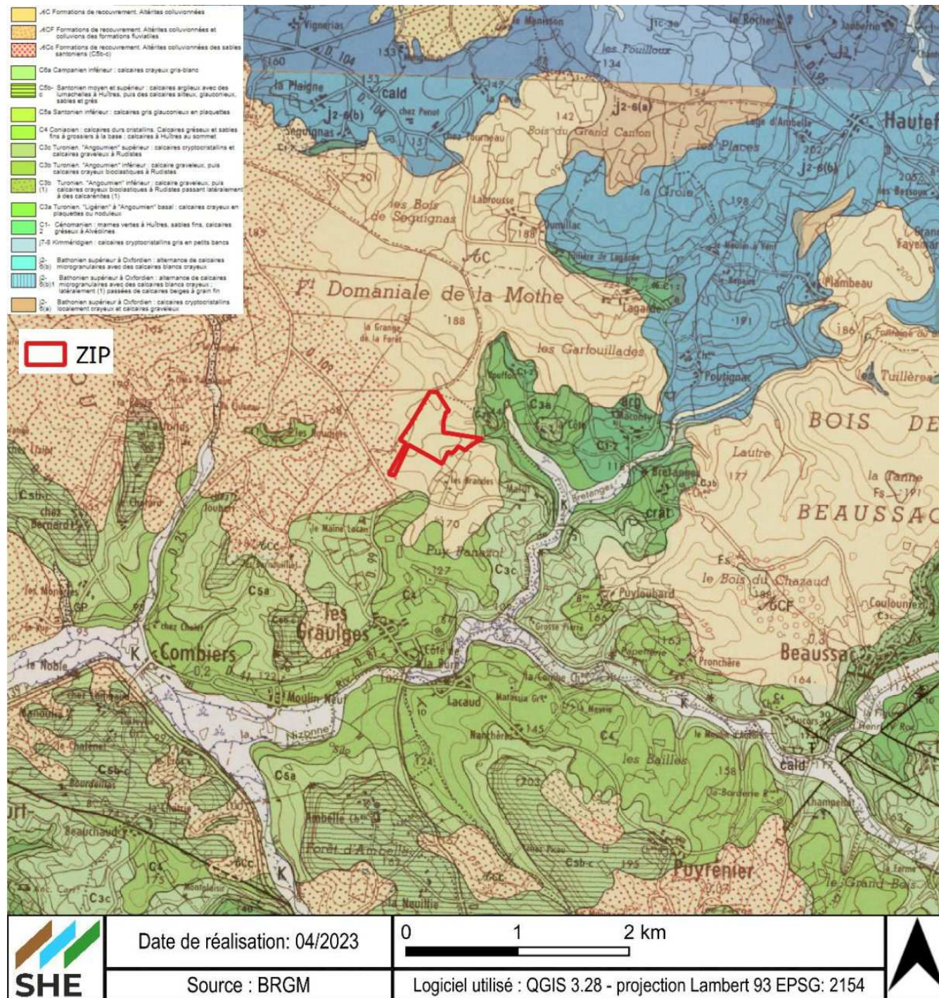
Figure 26 : Carte géologique
