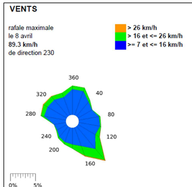
Illustration 17 : Rose des vents – Station de Coulounieix – Année 2022 – Source : Météo-France
