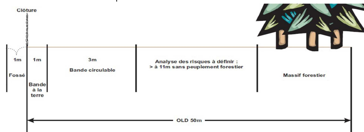
Figure 79 : Principe d'aménagement périphérique du site – Source : « Préconisations pour les parcs photovoltaïques au sol – SDIS 24 - 2022 »
